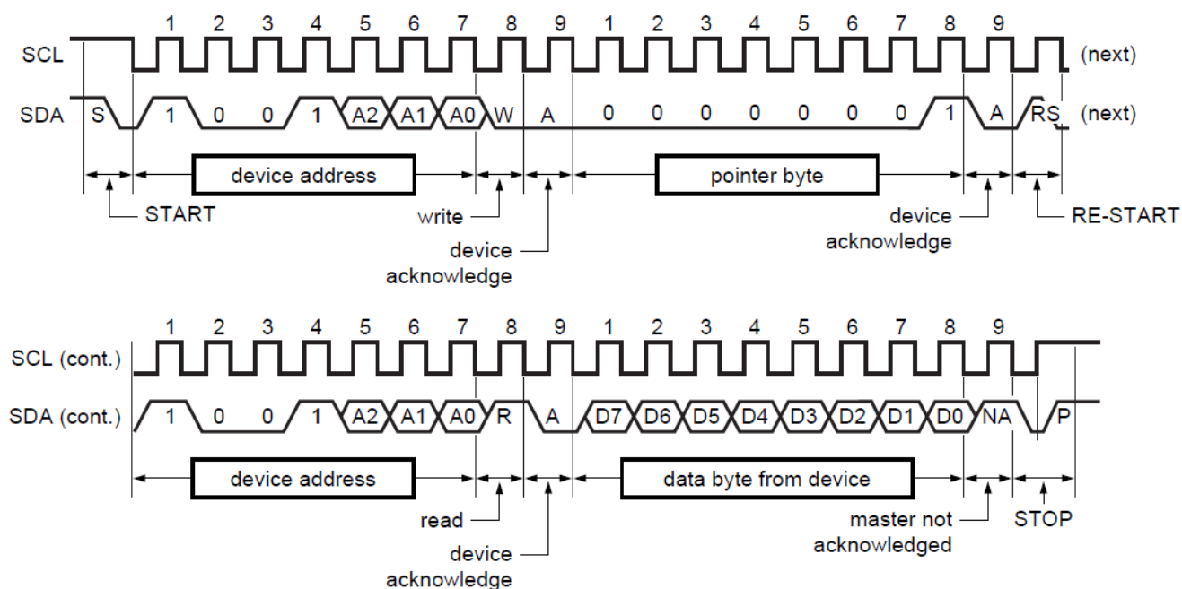
图 8.读取配置寄存器 (1-byte data)
