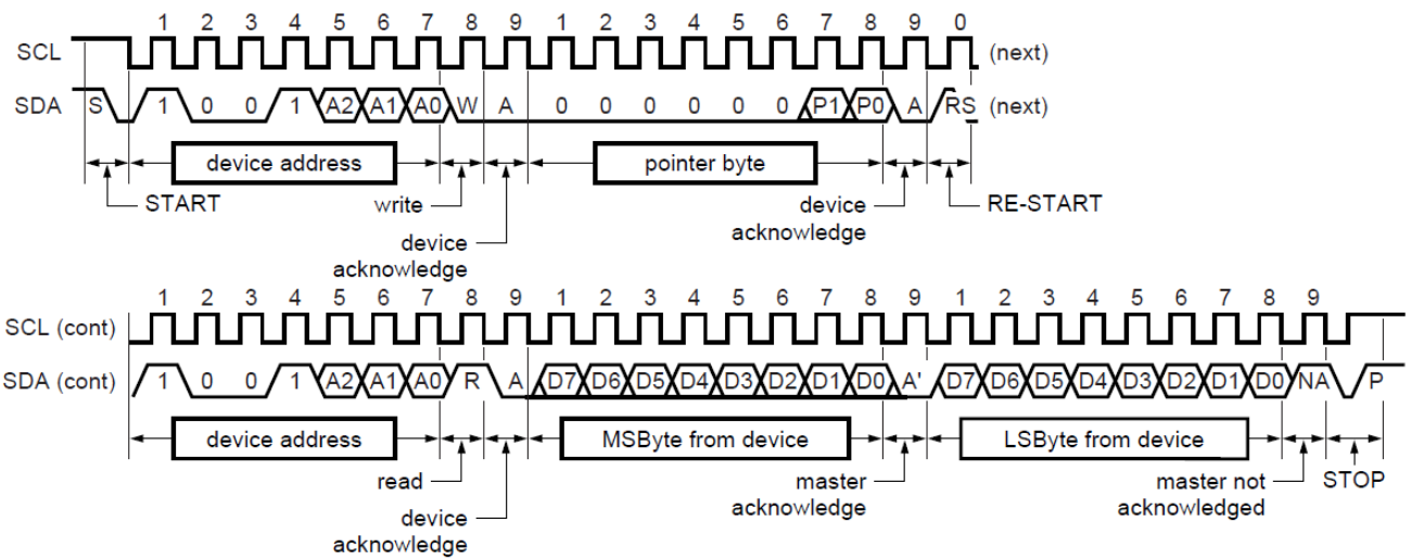
图 11. 读取温度，Tos 或 Thyst 寄存器 (2-byte data)
