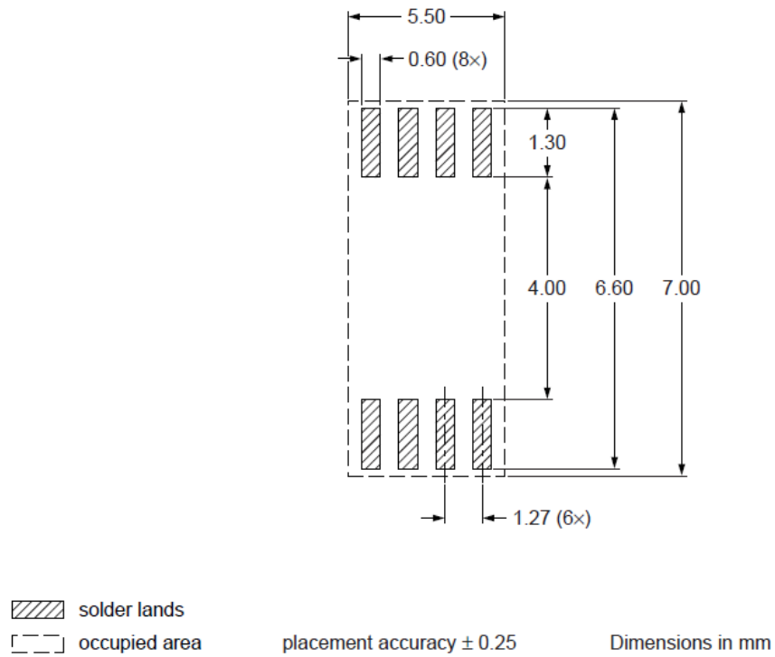
图 23. SOP8 PCB 引脚尺寸图
