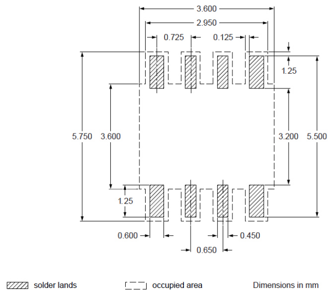
图 24. MSOP8/TSSOP8 PCB 引脚尺寸
