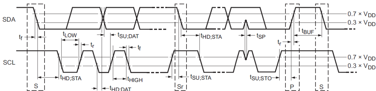
图 20. 时序图
